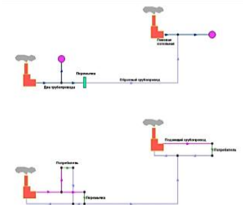
Рисунок19 - Подключение пикового источника. Вверху – однолинейное изображение сети, внизу – внутреннее представление
