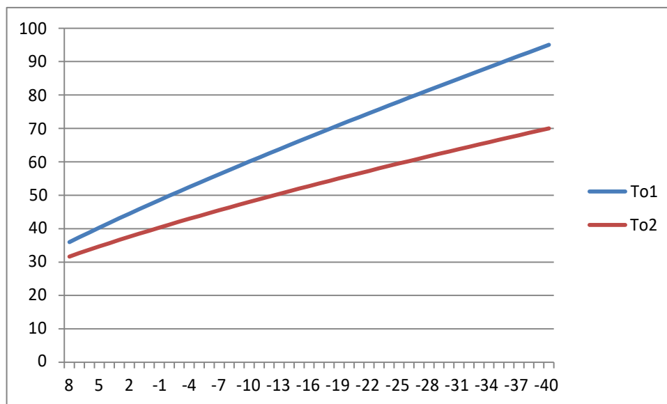
Рисунок 5-Температурный график тепловой сети
