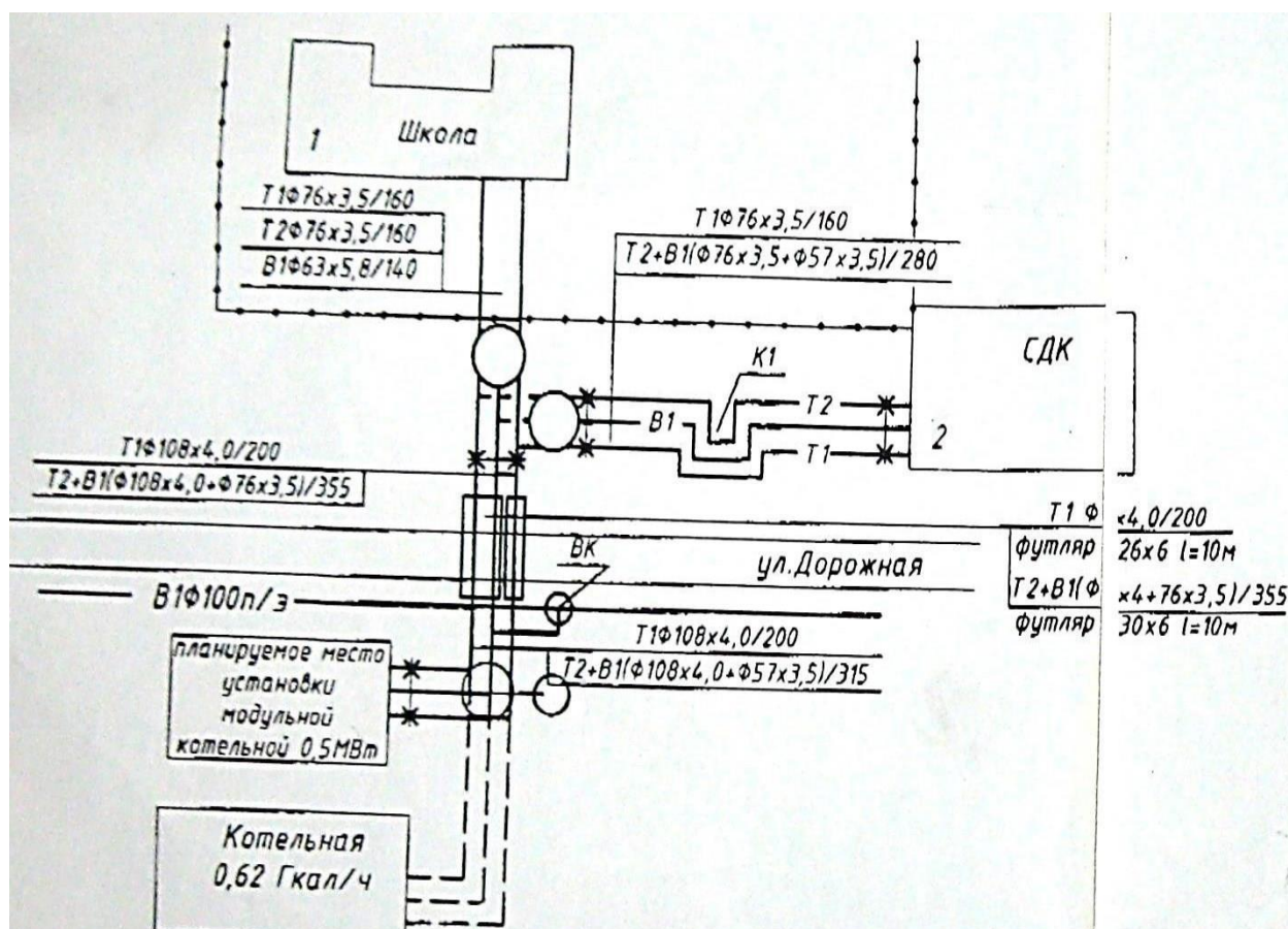
Рисунок 4 - Схема централизованного теплоснабжения от котельной с. Воробьево
