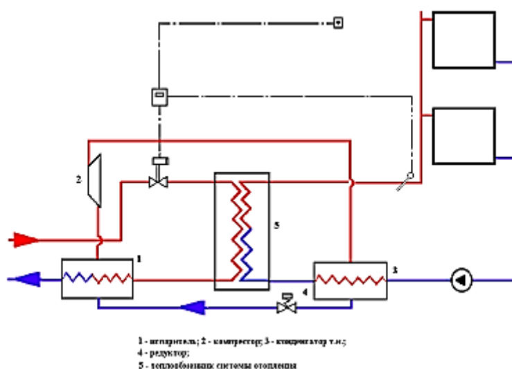
Рисунок47 - Схема теплового пункта с тепловым насосом и конденсатором на обратном трубопроводе системы отопления
