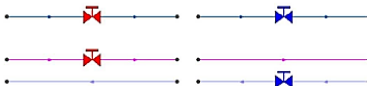
Рисунок37 - Однолинейное изображение (слева) и внутреннее представление (справа) сети с регуляторами давления
