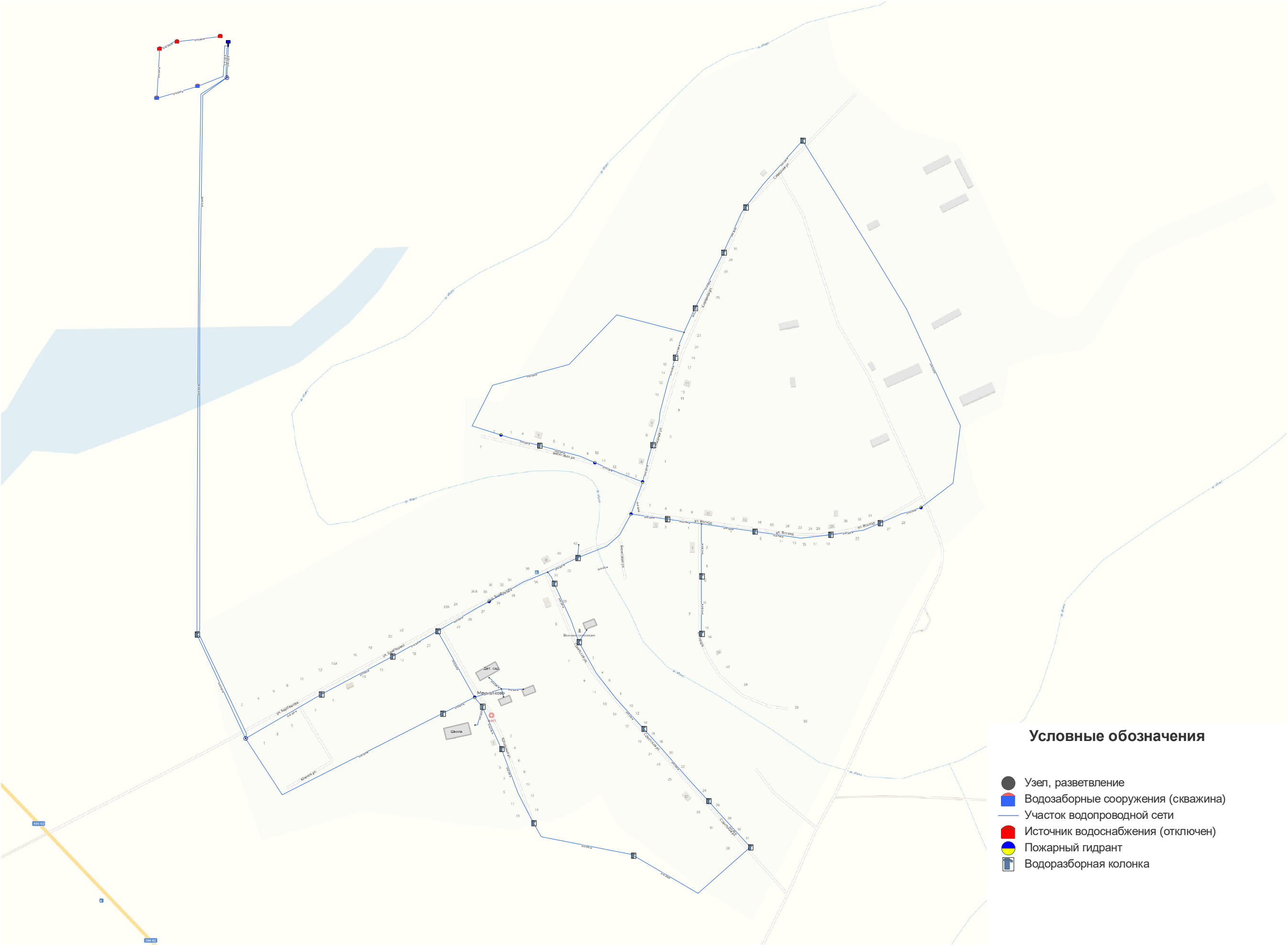
Приложение 1 - Схема сетей водоснабжения с. Меньшиков
