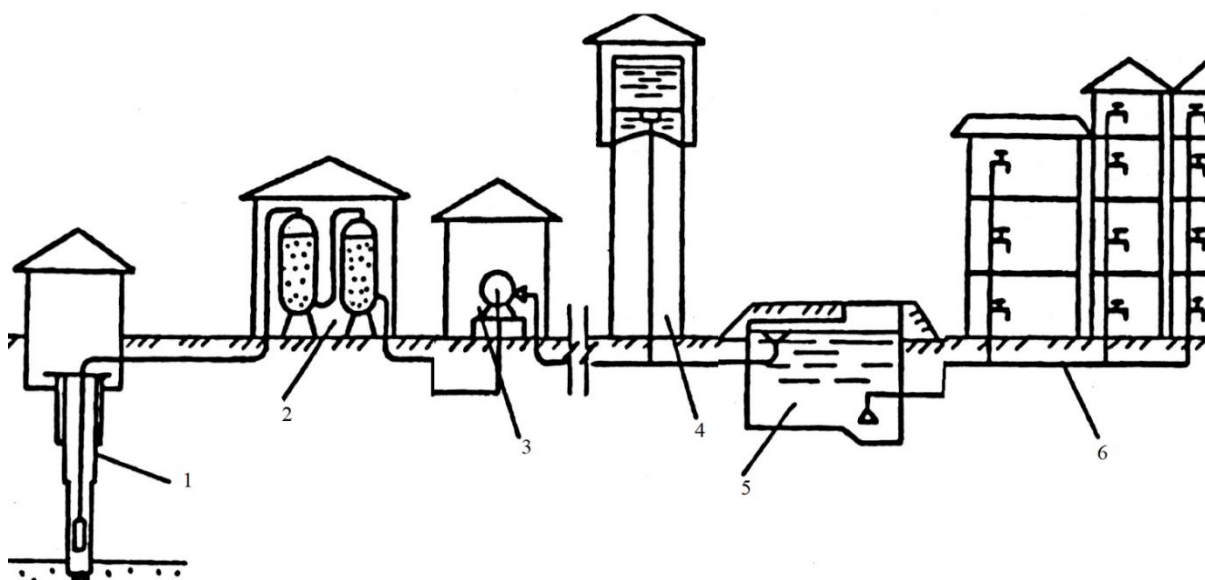
Рисунок 1 - Принципиальная схема водоснабжения поселения (1 – источник водоснабжения, скважина; 2 – резервуары чистой воды; 3 – насосная станция II-го подъема; 4 – водонапорная башня; 5 – блочно-модульная установка водоподготовки; 6 - потребители)
