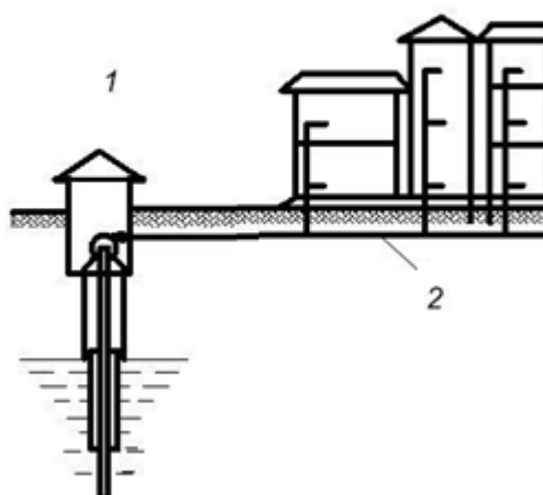
Рисунок 2 – Принципиальная схема водоснабжения п. Зыково, д. Игнатьевка, с. Старый Тартас (1 – источник водоснабжения, скважина; 2 – потребители)
