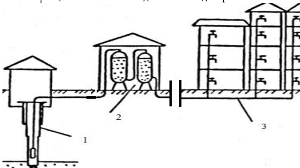
Рисунок 2 – Принципиальная схема водоснабжения с. Сибирцево 1-с (1 – источник водоснабжения, скважина; 2 – станция водоподготовки; 3 – потребители)
