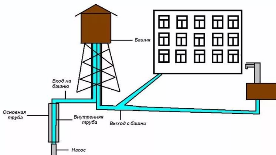
Рисунок 1 - Принципиальная схема водоснабжения д. Серп и Молот
