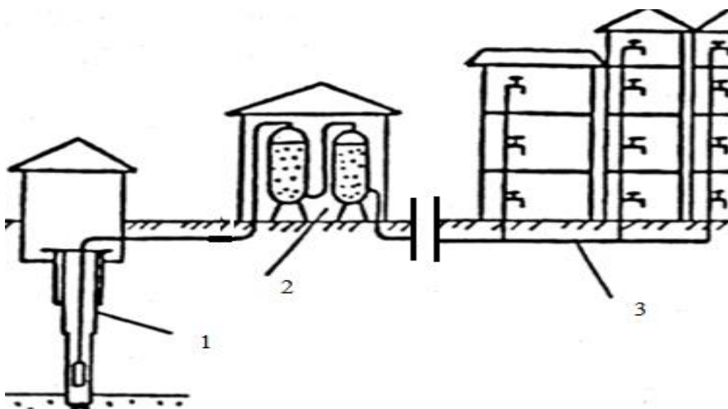
Рисунок 1 - Принципиальная схема водоснабжения с. Сибирцево 2-е (1 – источник водоснабжения, скважина; 2 – резервуар чистой воды; 3 – потребители)
