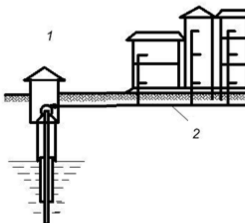
Рисунок 2 – Принципиальная схема водоснабжения д. Георгиевка (1 – источник водоснабжения, скважина; 2 – потребители)
