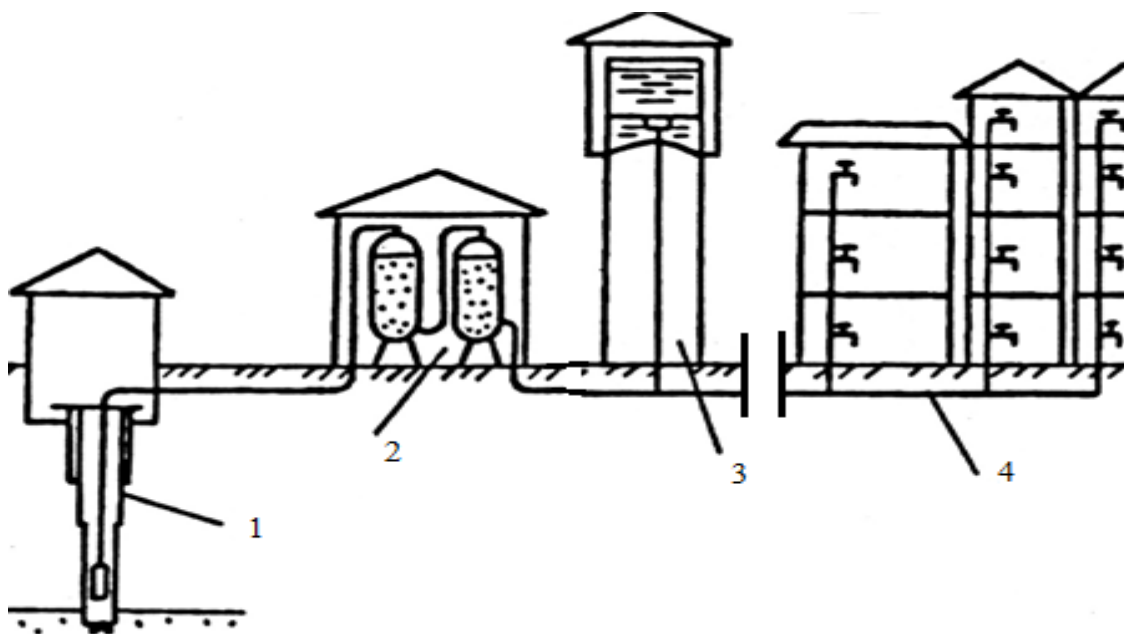
Рисунок 1 - Принципиальная схема водоснабжения с. Туруновка (1 – источник водоснабжения, скважина; 2 – резервуар чистой воды; 3 – водонапорная башня; 4 – потребители)
