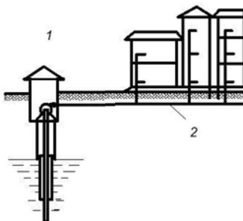
Рисунок 2 – Принципиальная схема водоснабжения д. Мариинка (1 – источник водоснабжения, скважина; 2 – потребители)
