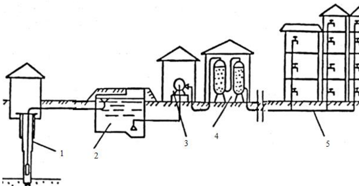
Рисунок 1 - Принципиальная схема водоснабжения с. Урез (1 – источник водоснабжения, скважина; 2 – резервуар чистой воды; 3 – насосная станция II-го подъема; 4 – блок-модуль станции водоподготовки; 5 – потребители)
