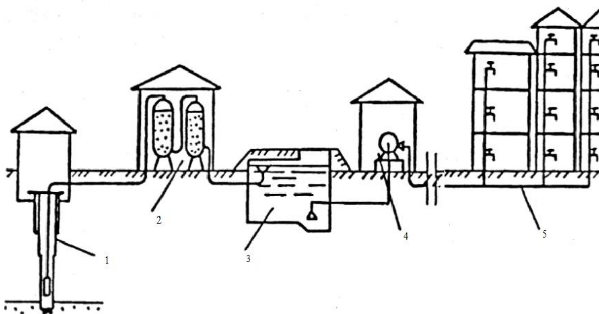
Рисунок 1 - Принципиальная схема водоснабжения поселения для водозабора, состоящего из 11-ти скважин (1 – источник водоснабжения, скважина; 2 – хлораторная; 3 – резервуары чистой воды; 4 – насосная станция II-го подъема; 5 – потребители)
