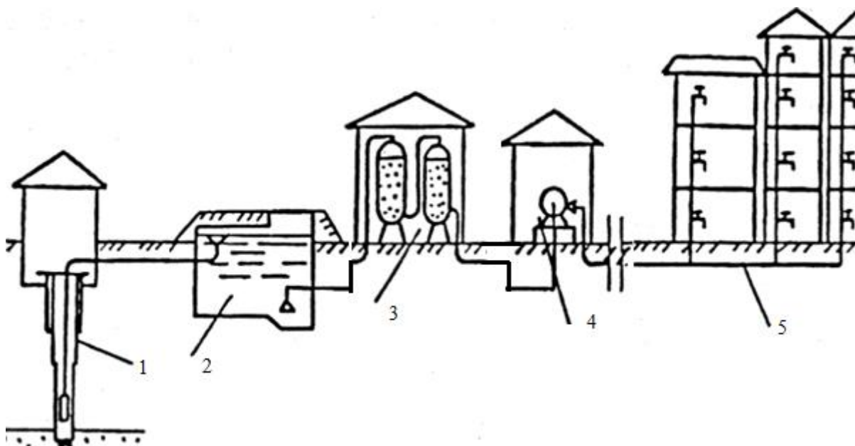
Рисунок 1 - Принципиальная схема водоснабжения с. Вознесенка (1 – источник водоснабжения, скважина; 2 – контррезервуар; 3 – УФ-стерилизатор; 4 – насосная станция II-го подъема; 5 – потребители)
