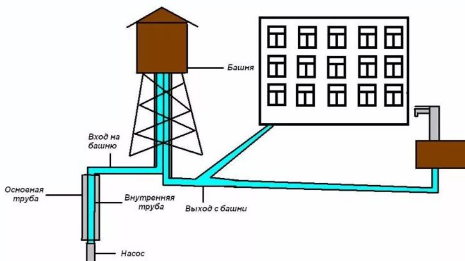
Рисунок 1 - Принципиальная схема водоснабжения с. Минино
